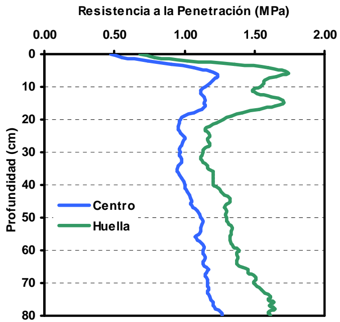
Fig. 6. Evaluación de la resistencia a la penetración en ensayos de rotaciones y fertilización de larga duración
